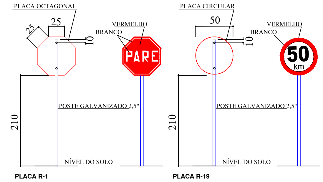
DETALHE PLACAS
