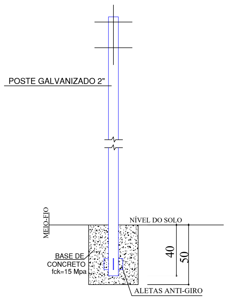
DETALHE FIXAÇÃO POSTE
